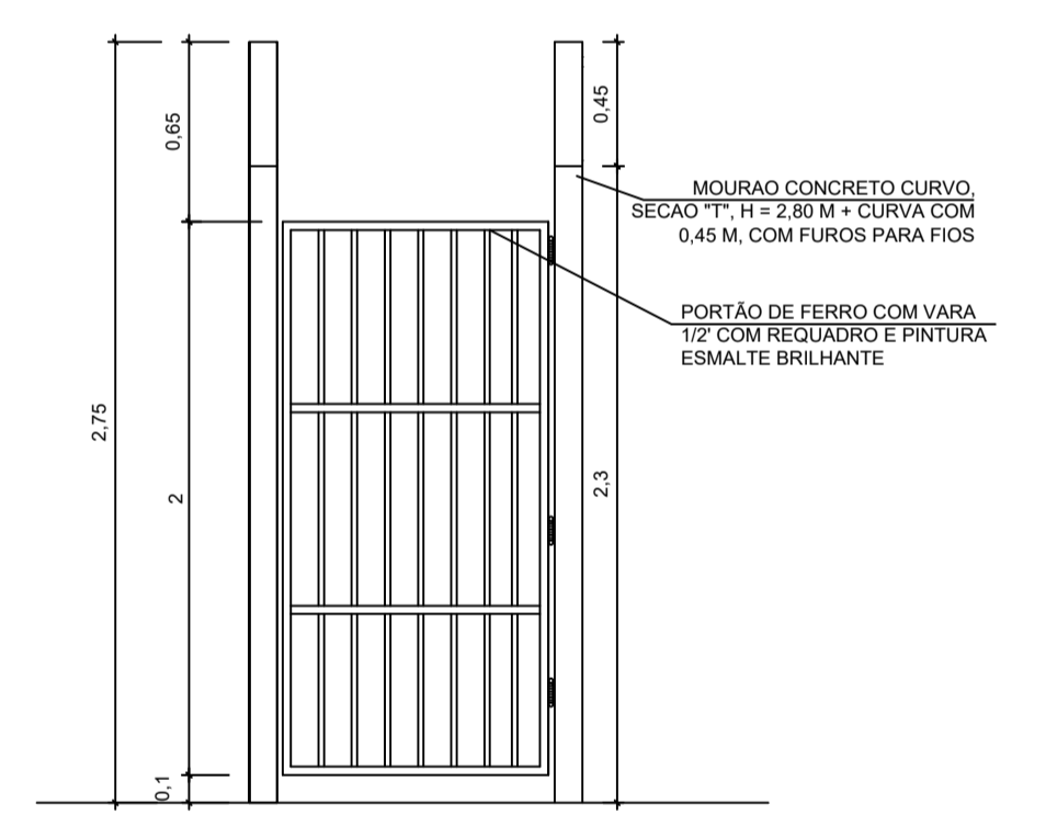
Det. Cerca Escala 1/30
