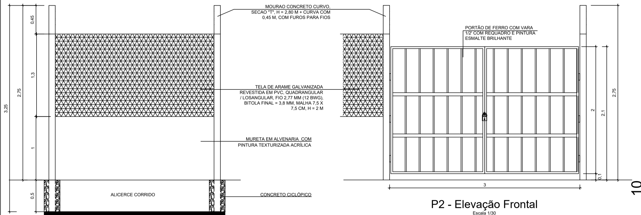
Det. Cerca Escala 1/30
